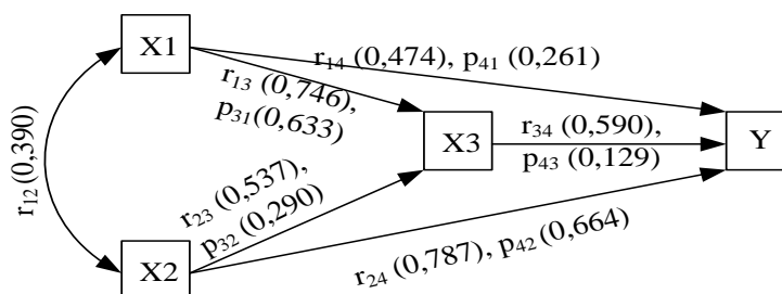
Gambar 2 Diagram Jalur dengan Nilai Koefisien Korelasi (r) dan Nilai Koefisien Jalur (p)
